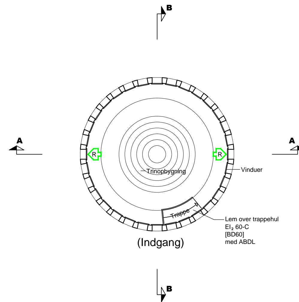
Plan 5 (udsigtsplatform) - Efter ombygning Mål 1:100
