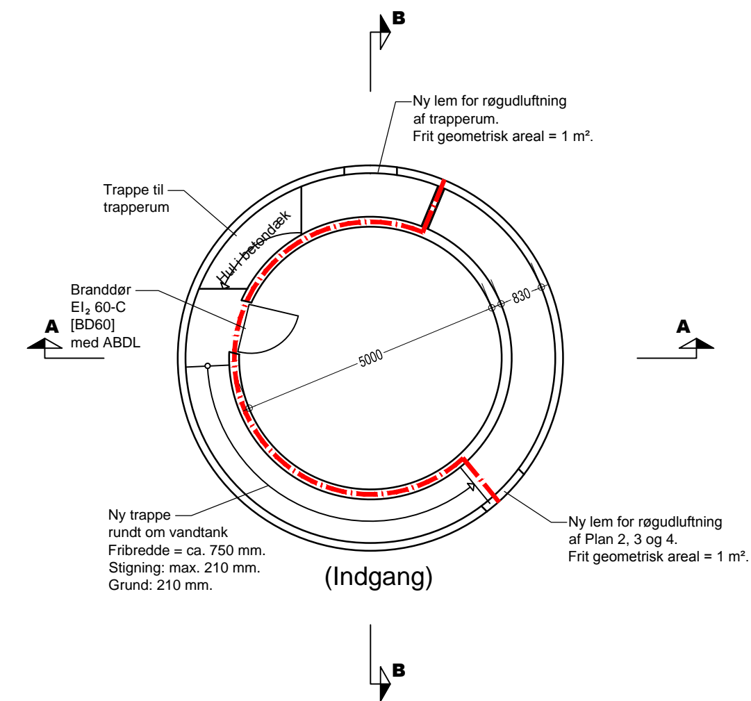
Plan 4 (vandtank) - Efter ombygning Mål 1:100
