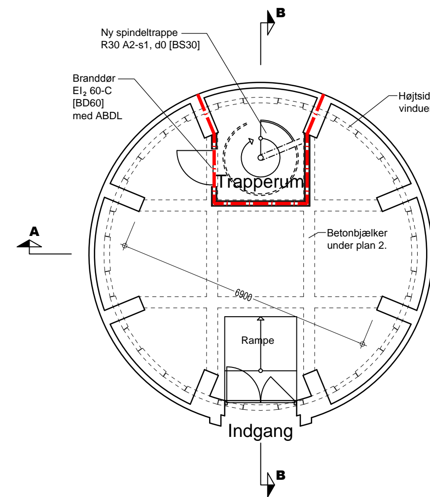
Plan 1 - Efter ombygning Mål 1:100
