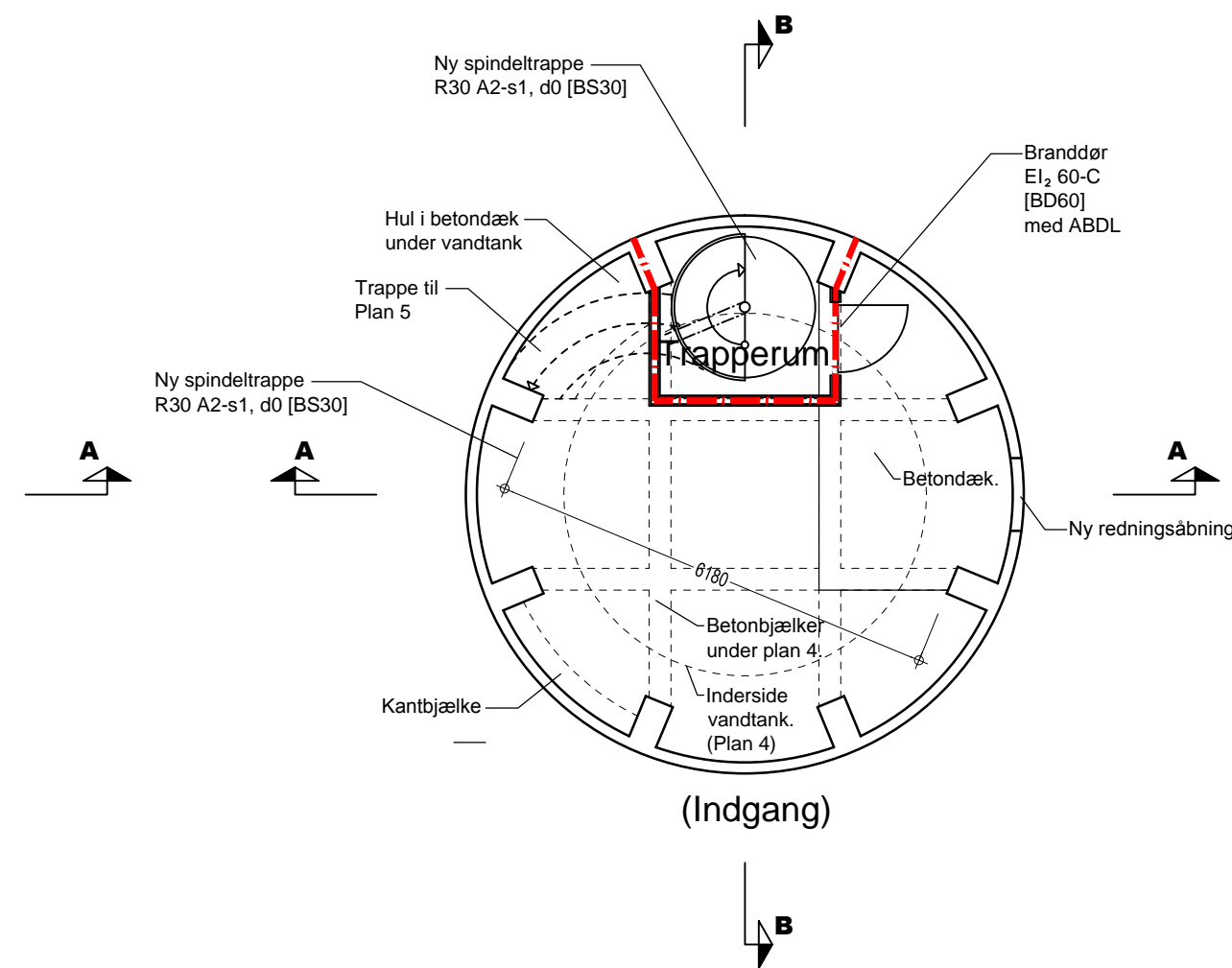
Plan 3 - Efter ombygning Mål 1:100
