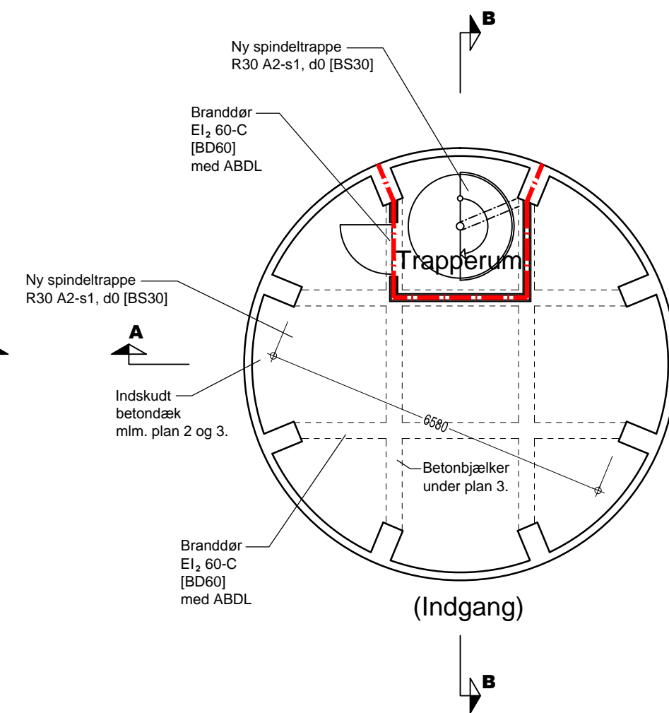
Plan 2 - Efter ombygning Mål 1:100
